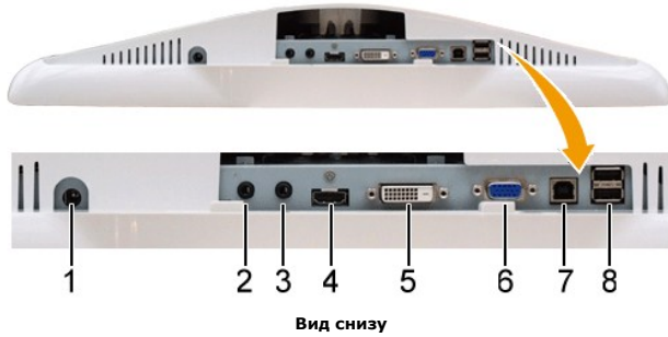
Вид снизу
